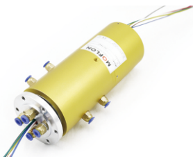
4 passages, M5
